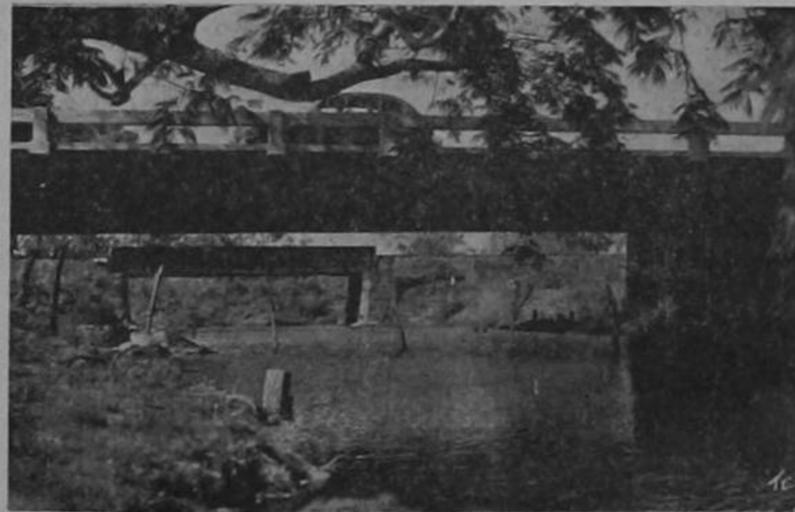
Puente sobre el Apanta, en el río del mismo nombre, de tres tramos de 16.40 metros de luz cada uno, construido en el Litoral N° 3 El Salvador, C. A.
